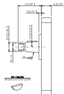
Type shaft 3-C9 Albero tipo 3-C9 Max torque / Coppia max: 250 Nm
