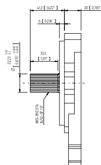
Type shaft SAEB-T13 Albero tipo SAEB-T13 Max torque / Coppia max: 450 Nm
