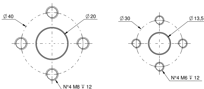
Type F / Tipo F
